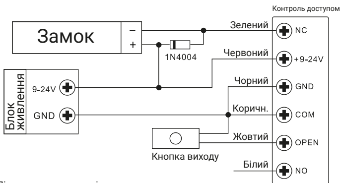
Підключення до магнітного замка
